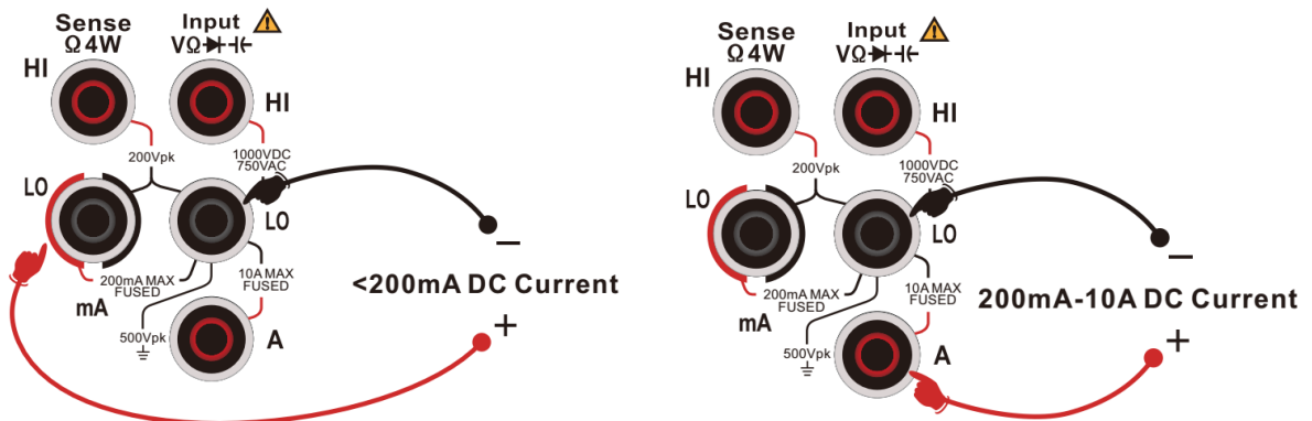
图 2-7 直流电流测量连接示意图
